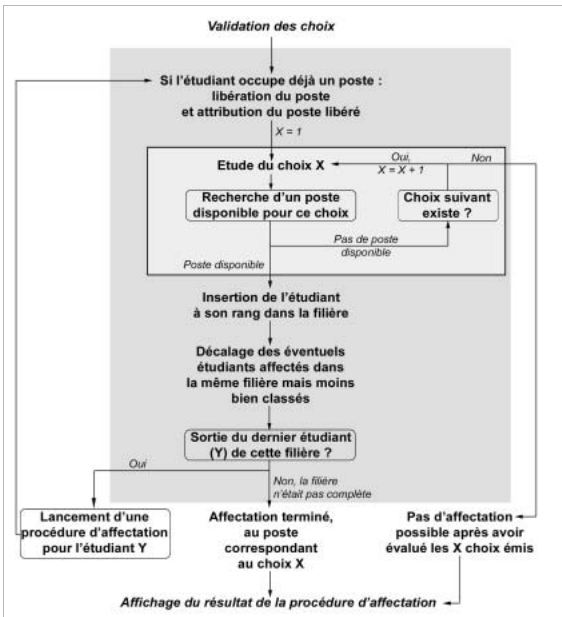
Figure 3 : Algorithme employé pour l'affectation d'un étudiant
