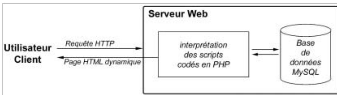
Figure 2 : Fonctionnement d'un serveur Web dynamique PHP / MySQL
